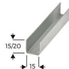
90P01 15x15x15 mm, th. 1,2 mm
